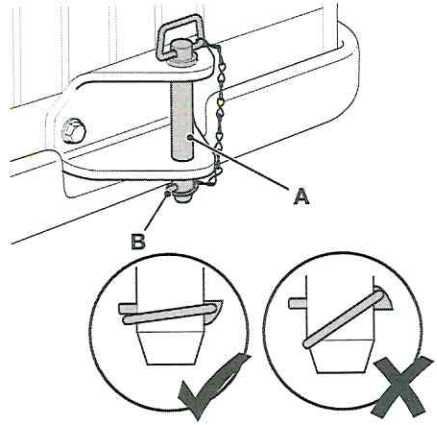
F-78. Instalación típica
