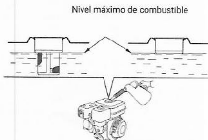
Imagen 10: Nivel máximo de combustible.
