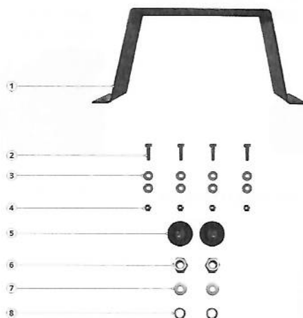
Imagen 22: Lista de materiales del Kit 3: Soporte
