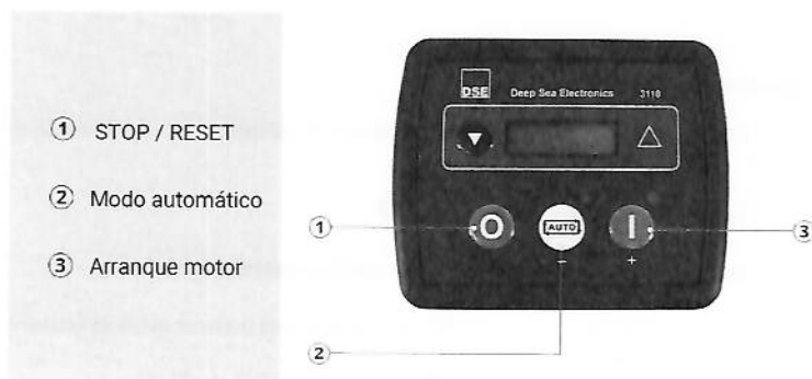
Imagen 12: Disposición modos de operación placa de control DSE 3110.
