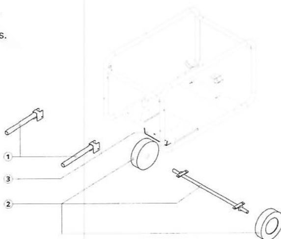
Imagen 18: Componentes del Kit transporte Dagartech
