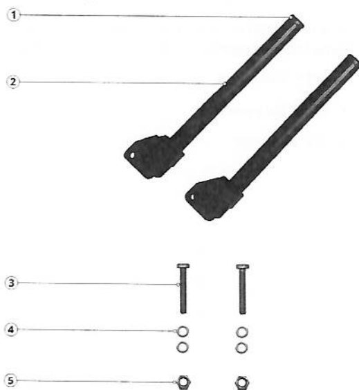
Imagen 19: Lista de materiales del Kit 1: Manerales.
