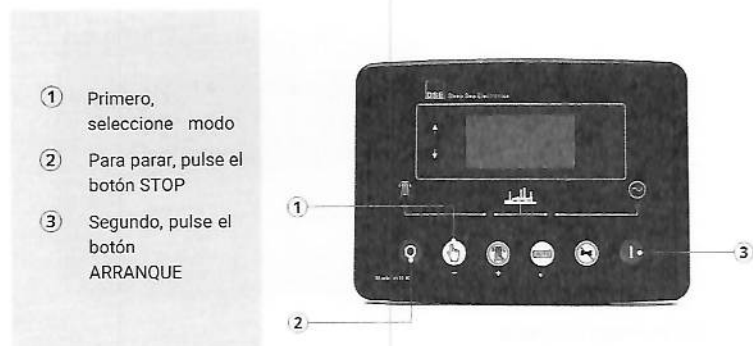
Imagen 13. Disposición modos de operación placa de control DSE 6020.
