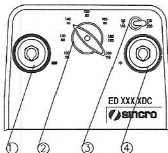
Imagen 17: Descripción del panel de la motosoldadora DGH 220 W DC.
