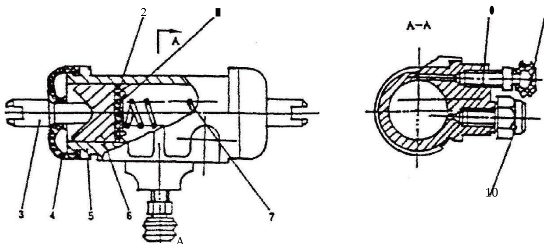
Cilindro esclavo de freno
