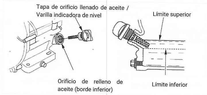
Imagen 9: Esquema componentes comprobación nivel de aceite.
