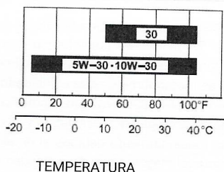
Imagen 8: Esquema temperatura-viscosidades aceite de motor.
