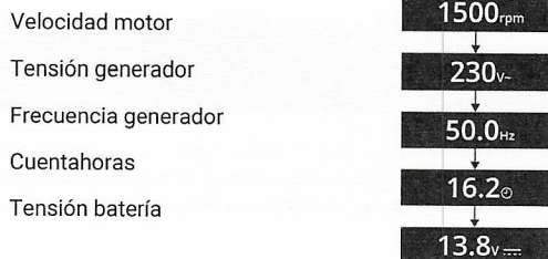
Imagen 11: Parámetros medibles en la placa de control DSE 3110.
