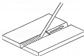
Imagen 15: Esquema buenas prácticas de soldadura con electrodo.
