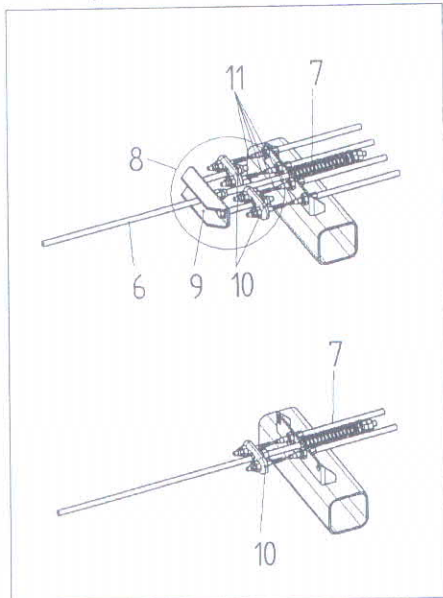
Figura 43 Dispositivo de transmisión para chasis en tandem y de un solo eje
