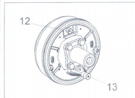
Figura 42 Freno de rueda KNOTT
