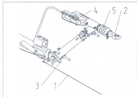
Figura 40 Dispositivo de tope de KNOTT
