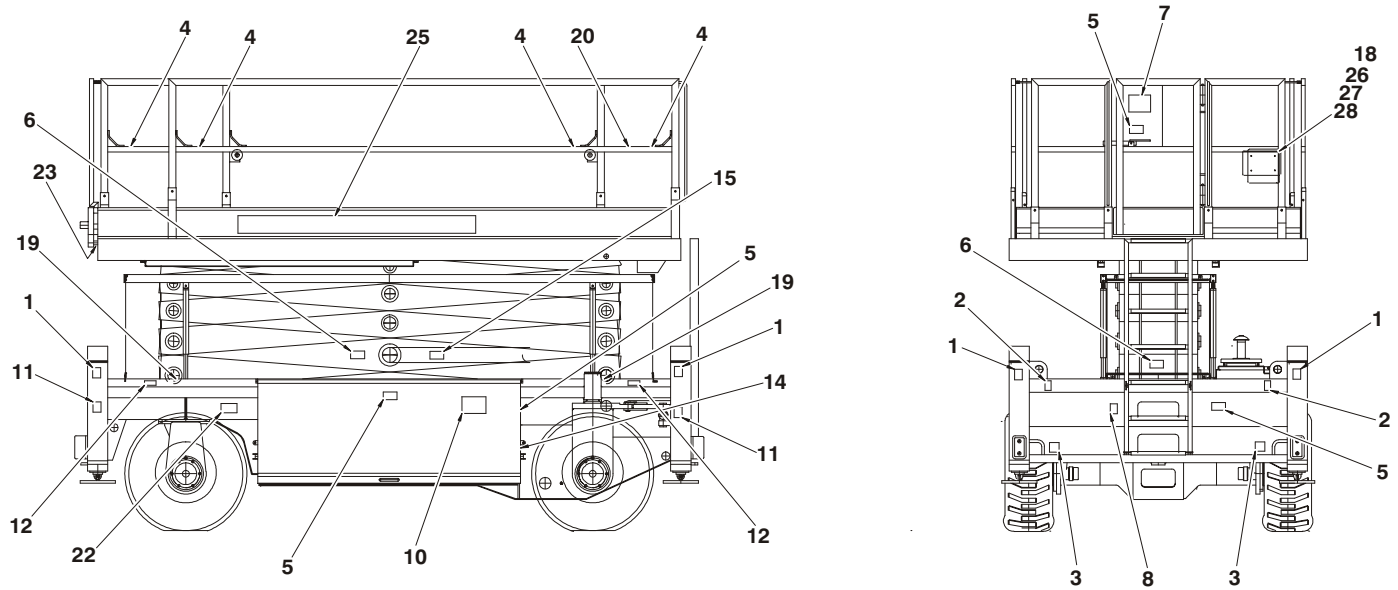
Figura 3-5. Ubicación de etiquetas - Hoja 1 de 2
