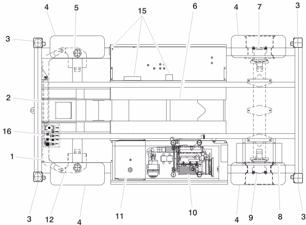
Figura 2-1. Diagrama de inspección visual diaria
