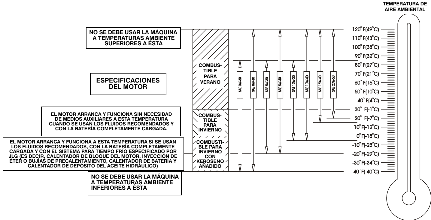
Figura 6-1. Especificaciones de temperatura de funcionamiento del motor - Hoja 1 de 2
