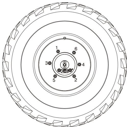
PATRÓN DE 6 TUERCAS
