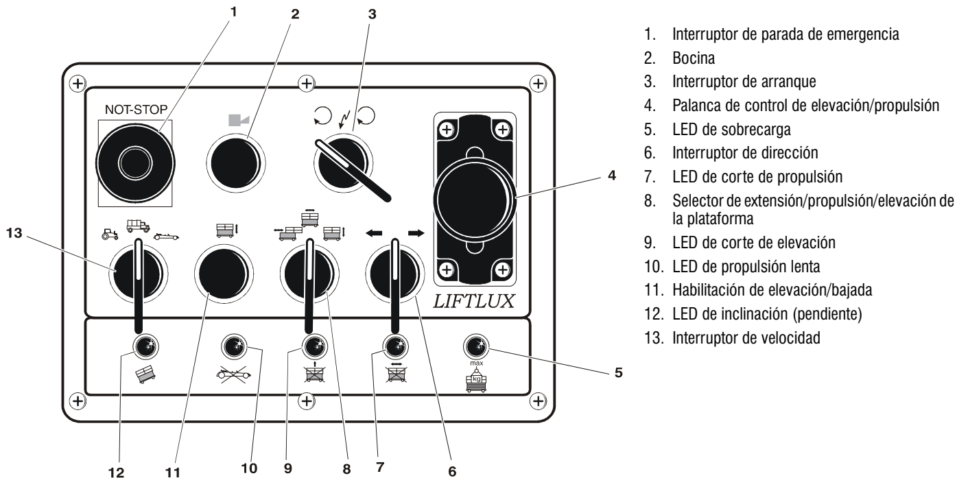
Figura 3-4. Puesto de controles de plataforma
