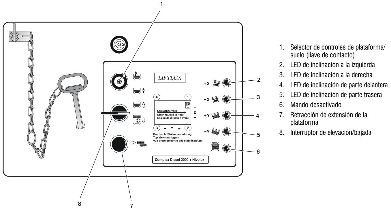
Figura 3-2. Control de plataforma/suelo
