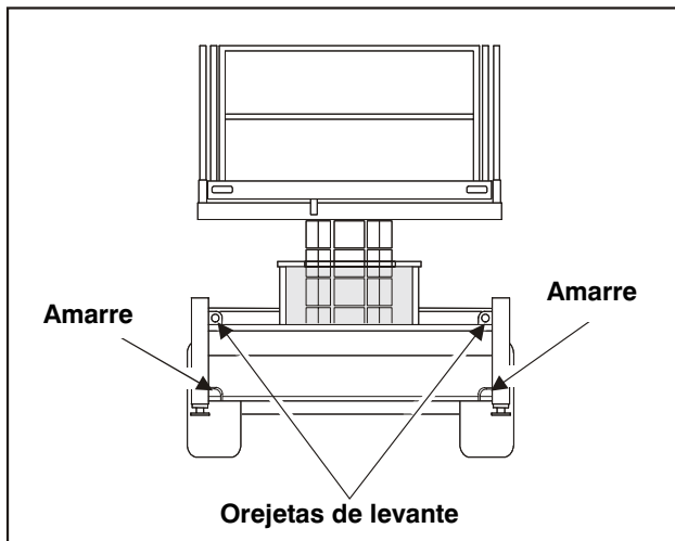
Figura 4-1. Ubicación de puntos de levante y amarre
