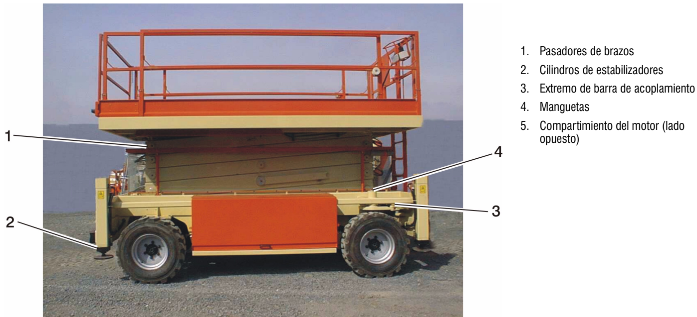
Figura 6-3. Diagrama de mantenimiento y lubricación por parte del operador
